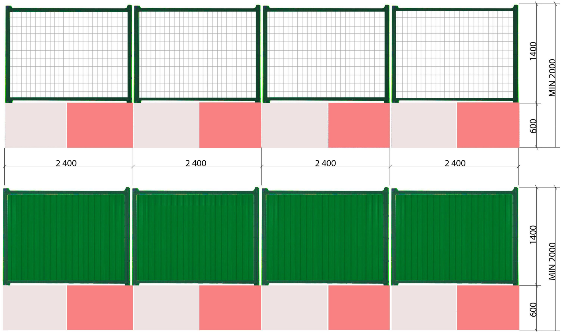
Проект ограждения строительной площадки
